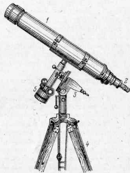
Рис. 18. Большой школьный рефрактор. 1 — тубус, 2 — окулярная часть, 3 — головка штатива, 4 — штатив, 5 — противовес
