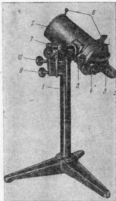
Рис. 17. Школьный меридиальный телескоп. 1 — штатив, 2 — труба телескопа, 3 — окуляр с увеличением 25, 4 — окуляр с увеличением 70, 5 — зенитная призма, 6 — визиры для наведения на избранный объект, 7—10 — винты зажима и винты тонкой наводки прибора
