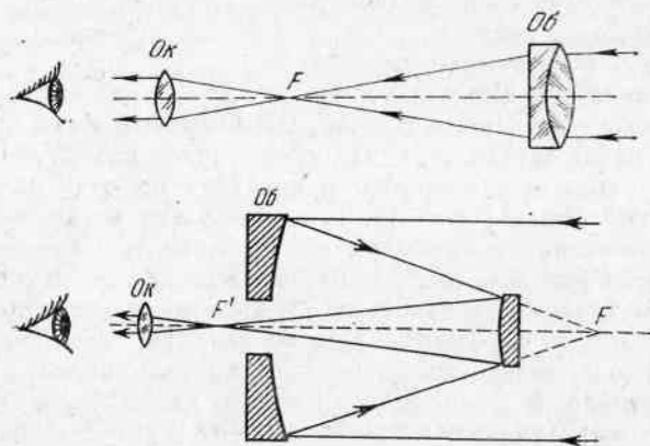
Рис. 14. Схемы рефрактора (вверху) и рефлектора. Об — объектив, Ок — окуляр, F — фокус
