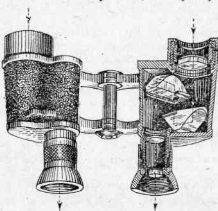
Рис. 12. Призмный бинокль
