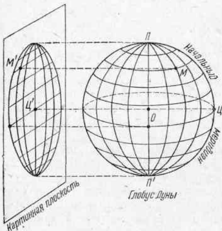
Рис. 81. Схема построения ортографической проекции полусферы
