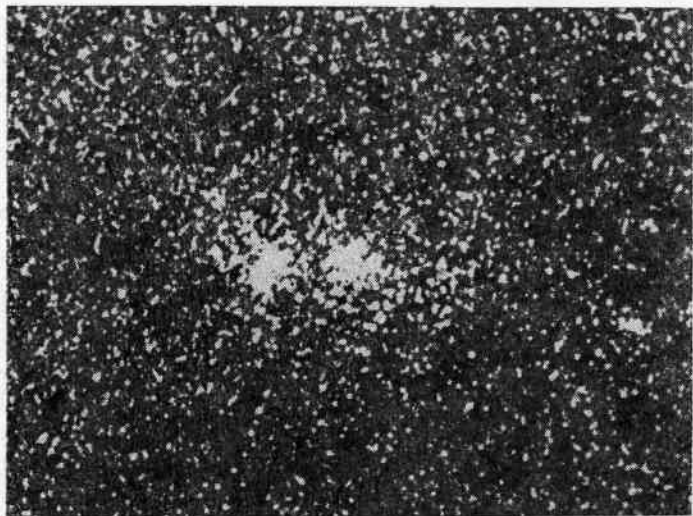
Рис. 42. Рассеянные звездные скопления \chi и \eta Персея
