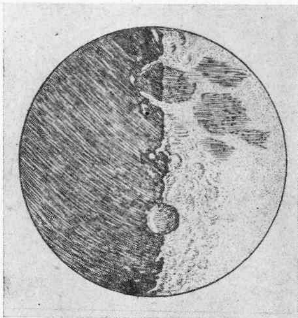
Рис. 76. Один из галилеевских рисунков Луны
