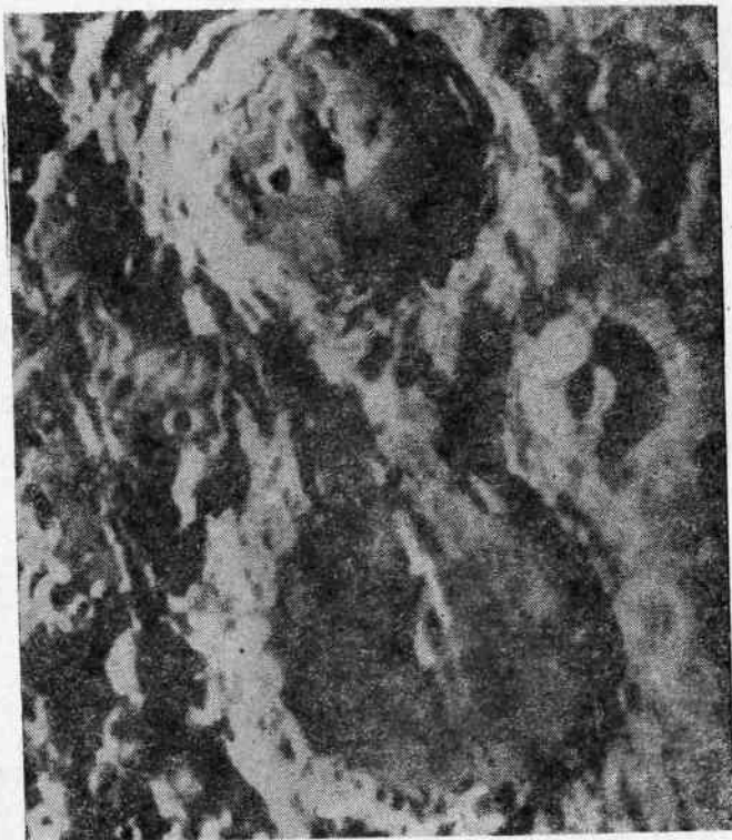
Рис. 95. Кратеры Альфонс (внизу), Арахель (вверху) и Альпетрагий (справа)
