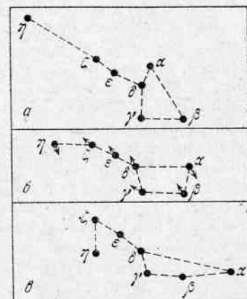
Рис. 31. Движения звезд Ковша Большой Медведицы: а — вид 100 000 лет назад, б — в настоящее время, в — через 100 000 лет
