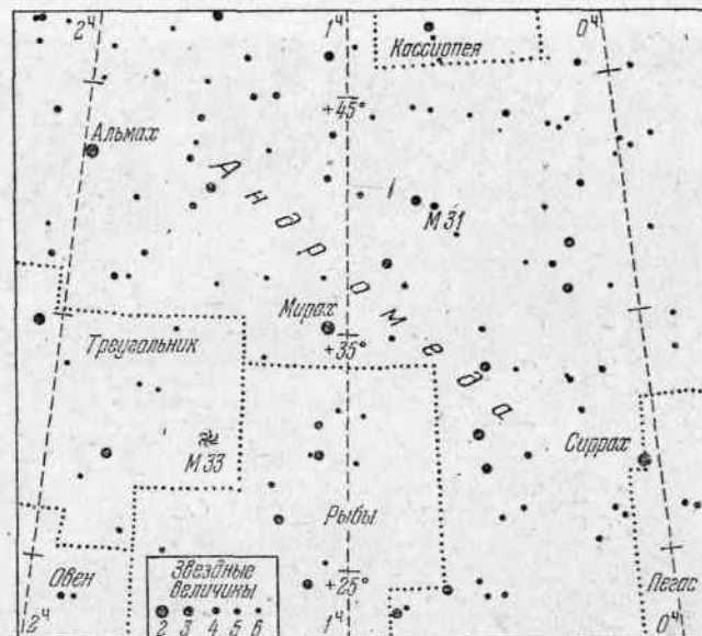
Рис. 44. Расположение на небе туманности М 33 в Треугольнике
