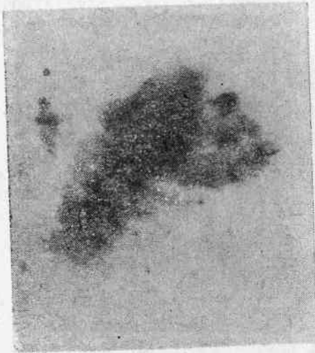
Рис. 10. Пекулярная галактика NGC 2685
