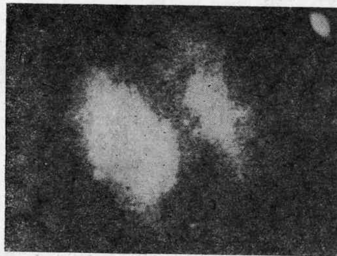
Рис. 68. Фотография части галактического ядра в инфракрасном диапазоне волн
