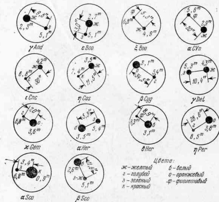
Рис. 106. Расположение и цвета некоторых двойных звезд
