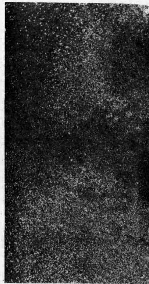
Рис. 67. Млечный Путь в окрестности созвездия Щита
