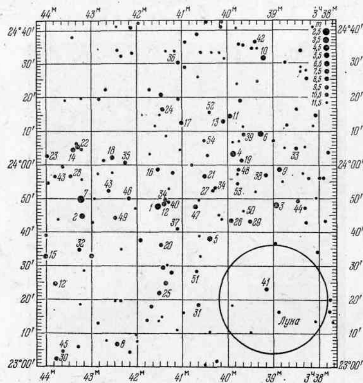
Рис. 50. Вид Плеяд в телескоп (кружком обозначены размеры лунного диска): 1 — Альциона, 2 — Атлас, 3 — Электра, 4 — Майя, 5 — Мeroпа, 6 — Тайгета, 7 — Плейона, 9 — Целена, 11 — Астеропа
