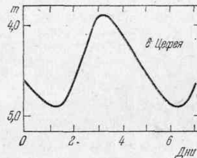
Рис. 36. Кривая блеска \delta Цефея
