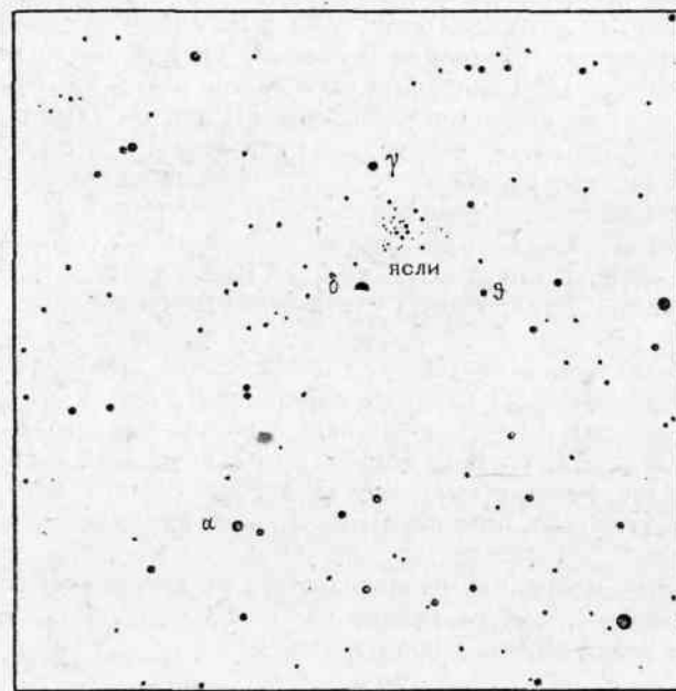
Рис. 60. Звездное скопление Ясли в созвездии Рака
