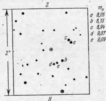
Рис. 38. Карта окрестностей переменной звезды RU Жи́рафа (отмечена кружком). Справа приведены звездные величины звезд сравнения
