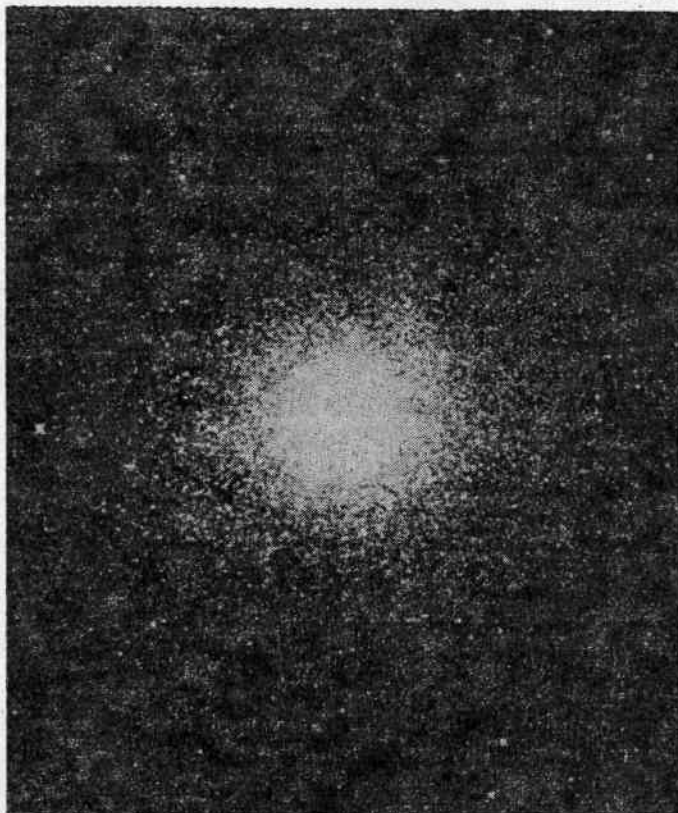
Рис. 64. Шаровое звездное скопление М 13
