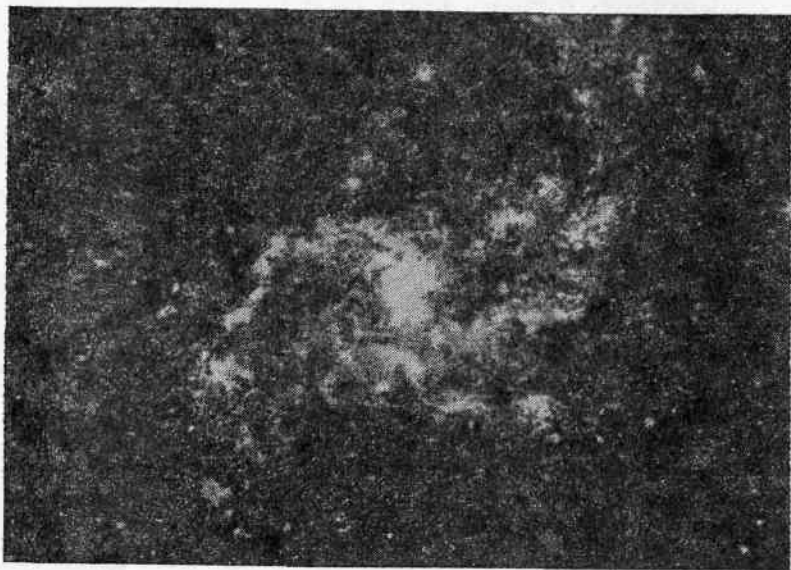
Рис. 45. Фотография галактики М 33
