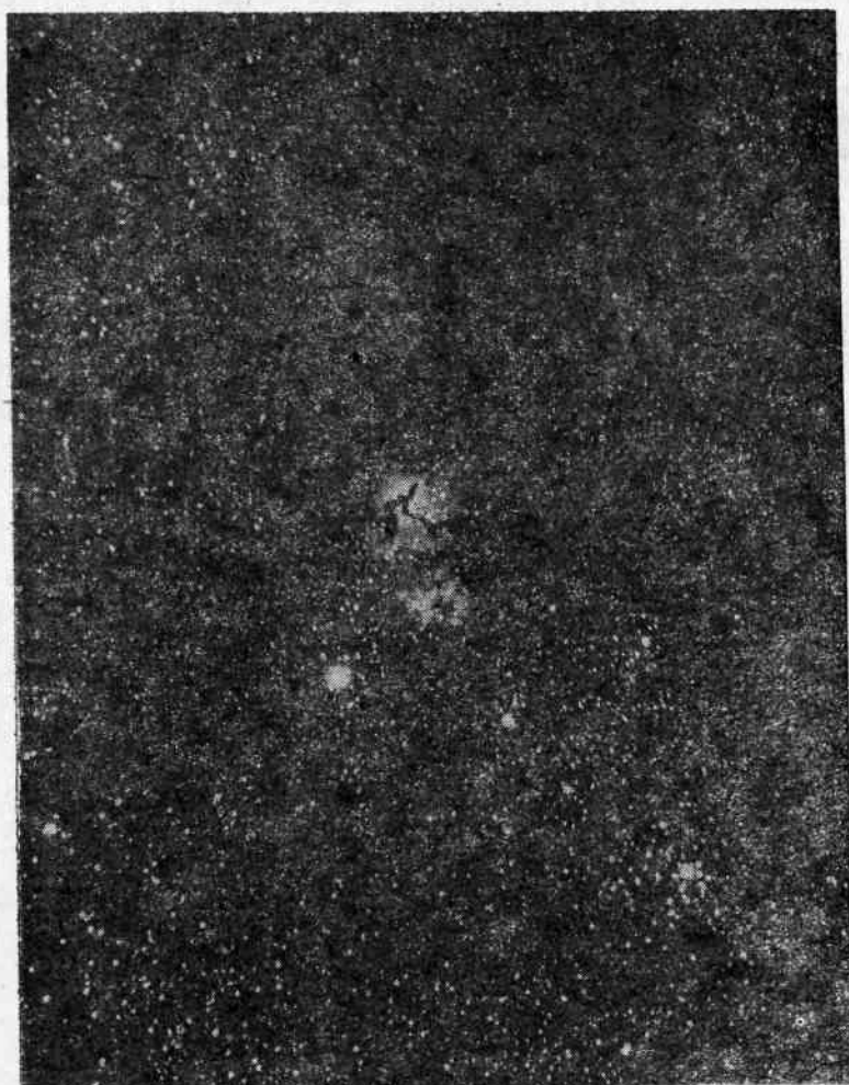
Рис. 69. Тройная туманность в созвездии Стрельца
