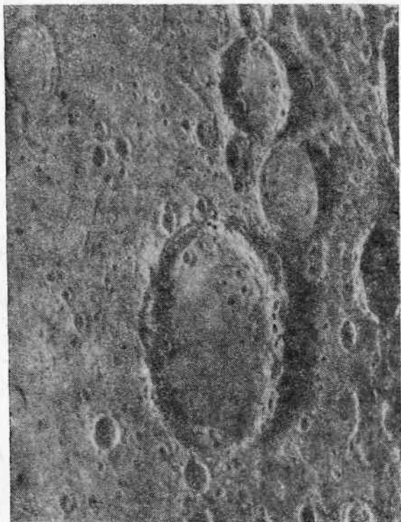
Рис. 97. Столовая гора Варгентин
