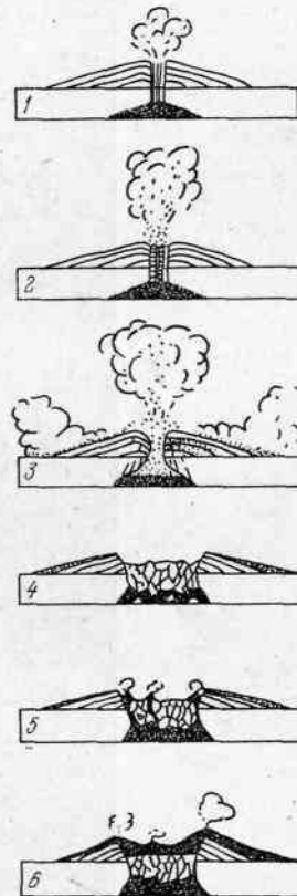
Рис. 84. Последовательные стадии образования кальдеры
