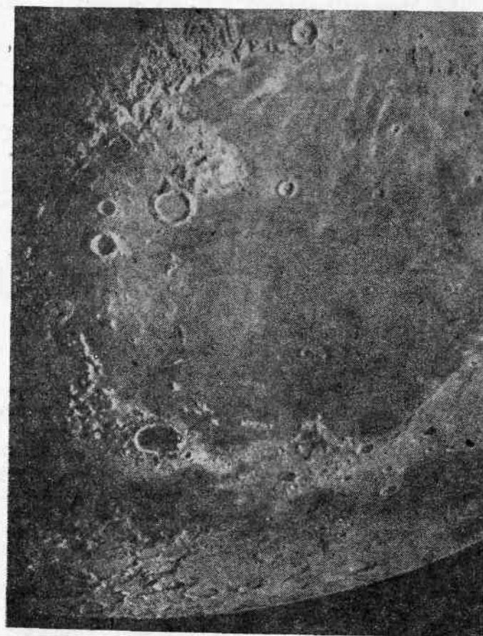
Рис. 90. Море Дождей и окаймляющие его горные хребты (изображение перевернутое)
