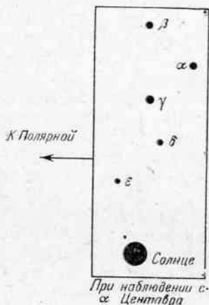
Рис. 73. Вид Солнца с α Центавра
