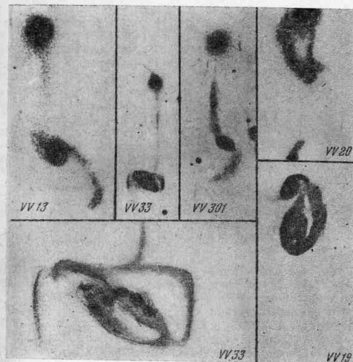
Рис. 9. Еще несколько систем взаимодействующих галактик
