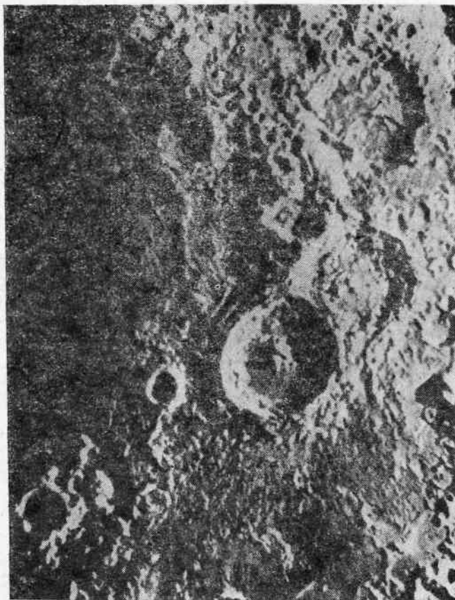
Рис. 89. Кратеры Теофил, Кирилл и Катарина
