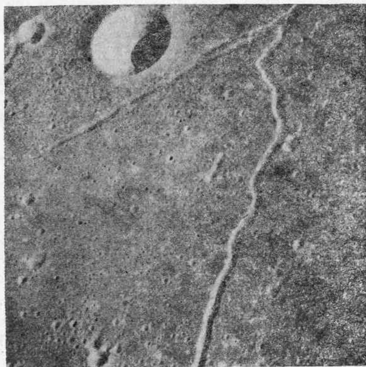
Рис. 105. Трещина Гиги (вверху) на видимом полушарии Луны и одна из лунных борозд (внизу), сфотографированная на обратной стороне Луны
