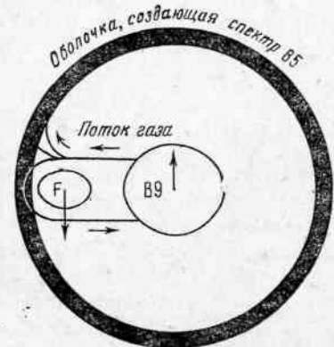
Рис. 62. Схема строения системы \beta Лиры
