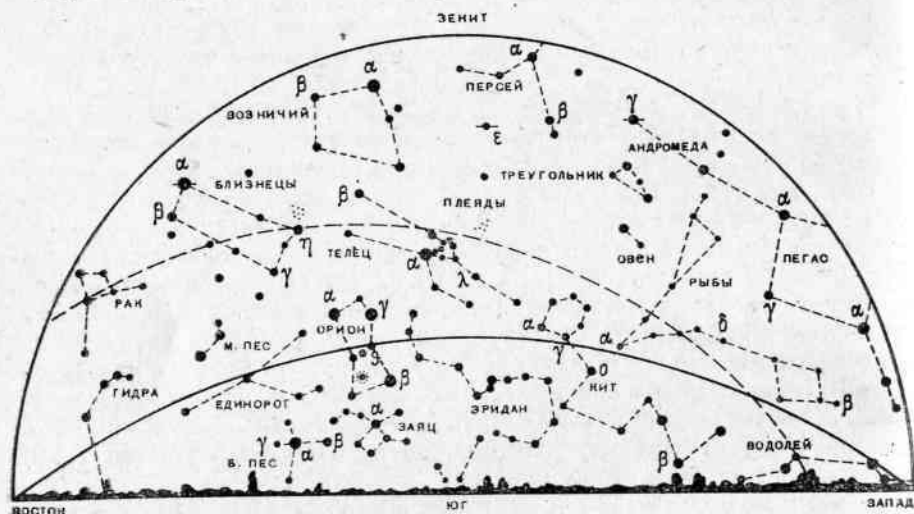
Рис. 48. Южная часть зимнего неба
