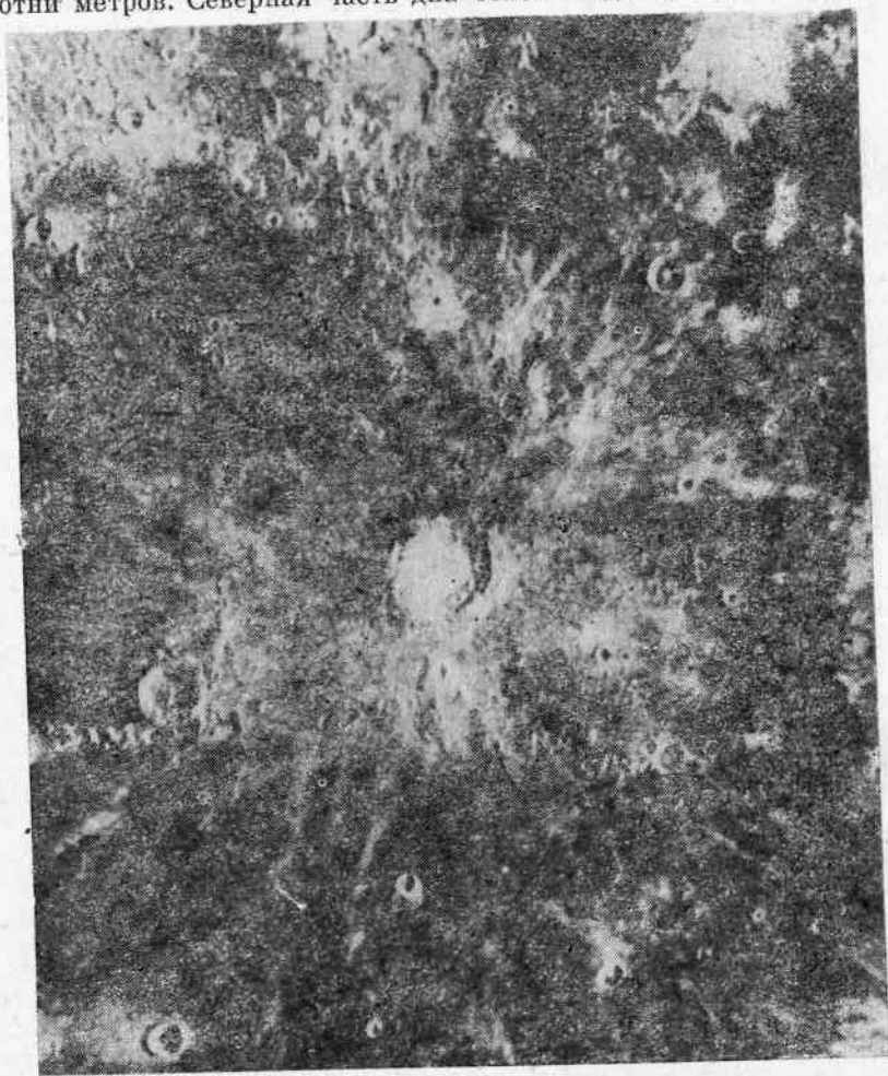
Рис. 93. Система светлых лучей кратера Коперник
