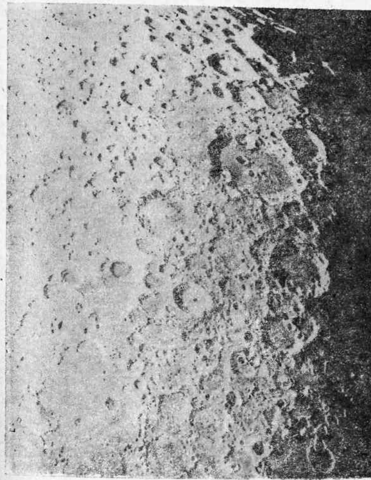
Рис. 80. Типичный лунный рельеф (область вблизи кратера Клавий)
