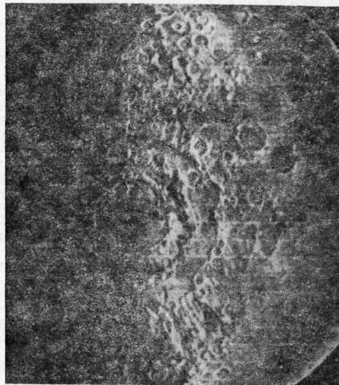
Рис. 104. Море Восточное и его окрестности
