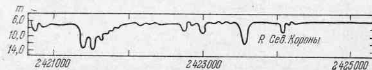
Рис. 65. Кривая блеска R Северной Короны
