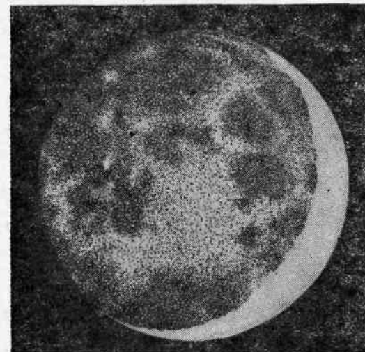
Рис. 82. Пепельный свет Луны
