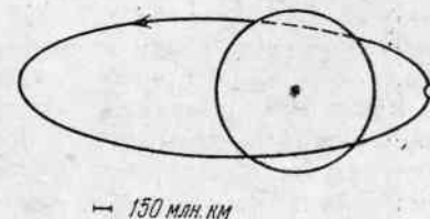
Рис. 56. Система \epsilon Возничего
