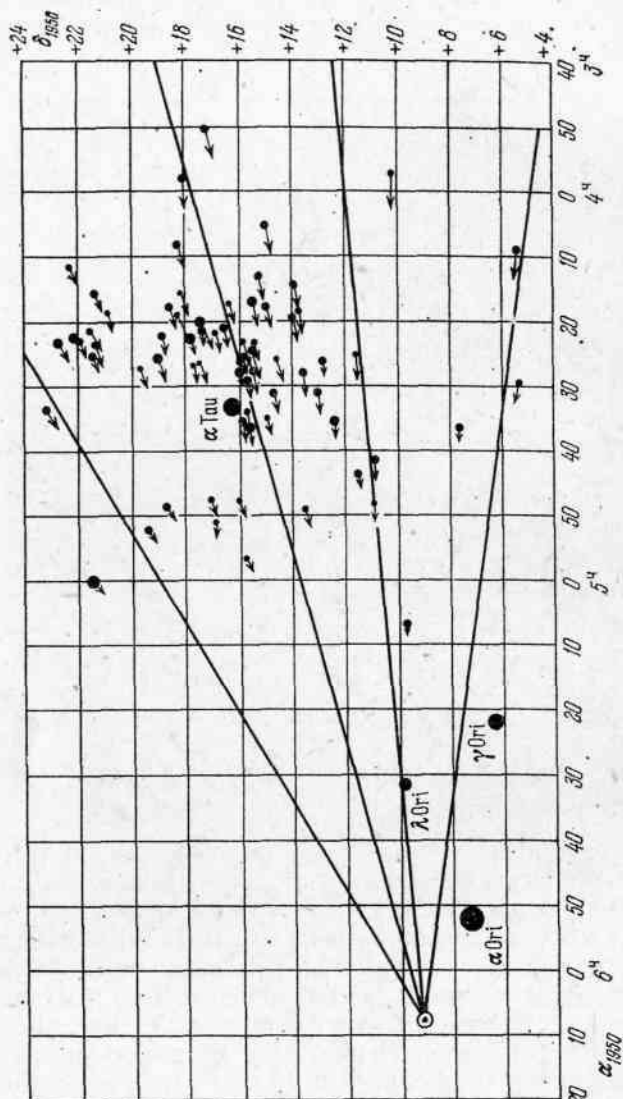
Рис. 53. Гиады и их собственные движения
