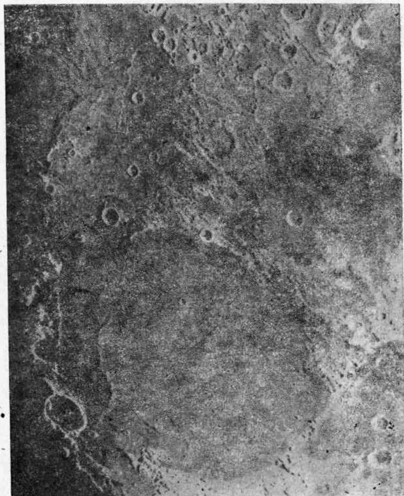
Рис. 87. Море Ясности и его окрестности
