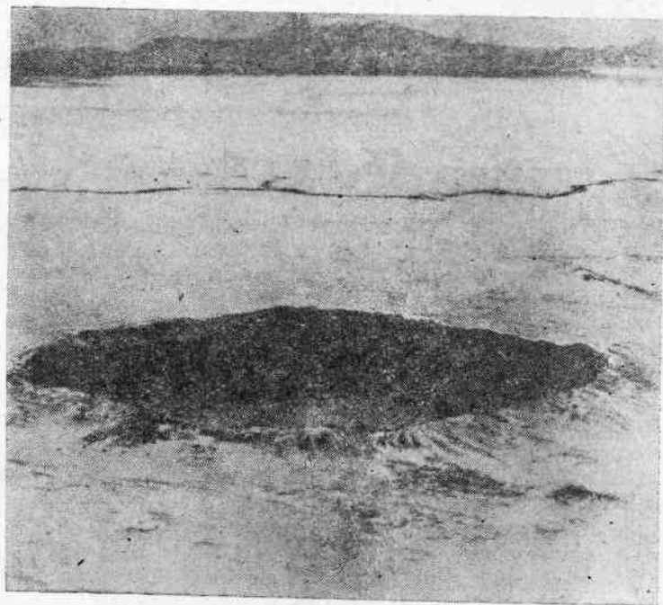
Рис. 83. Аризонский метеоритный кратер
