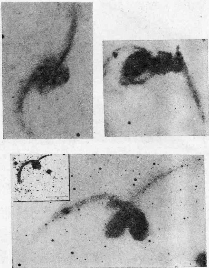
Рис. 8. Необычные галактики VV 79 (вверху слева), VV 243 — «Оса» (вверху справа) и VV 245 (внизу)
