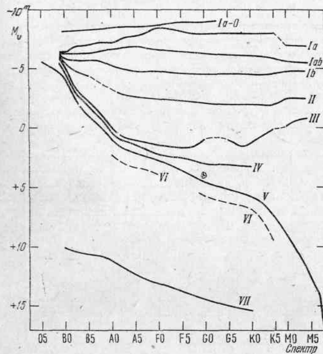
Рис. 3. Диаграмма Герцшпрунга — Рассела. Последовательности: Ia-0 — ярких сверхгигантов, Ia — ярких сверхгигантов, Iab — средних сверхгигантов, Ib — слабых сверхгигантов, II — ярких гигантов, III — слабых гигантов, IV — субгигантов, V — главная последовательность, VI — субкарликов, VII — белых карликов
