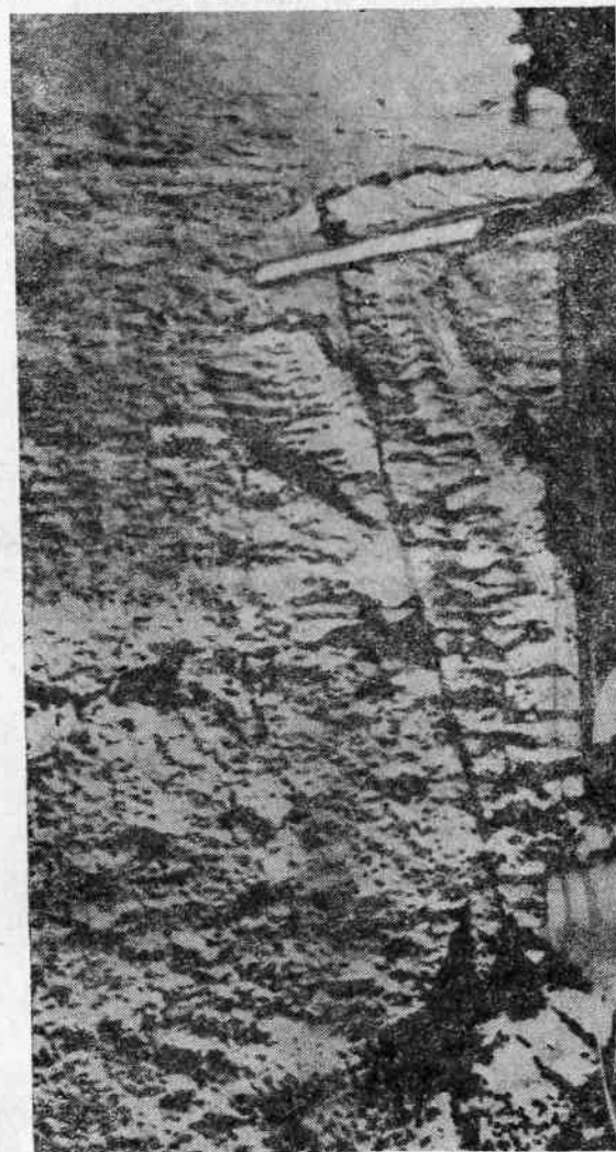
Рис. 101. Следы «Лунохода-1» на лунной поверхности
