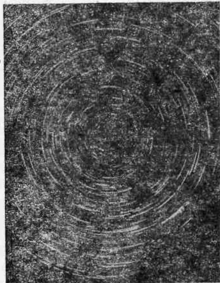
Рис. 21. Суточное движение звезд в околополярной области
