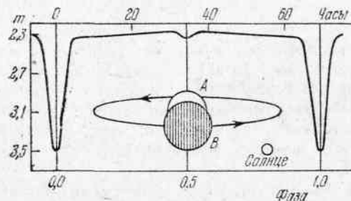
Рис. 41. Схема изменения блеска Алголя
